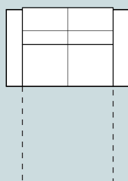
52 (P/L) – rozklad k dílům: 06, 07, 08 ložná plocha: 123 × 205/ v. 42
