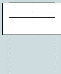
53 (P/L) – rozklad k dílům: 09, 10, 11 ložná plocha: 153 × 205/ v. 42
